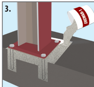
Процес на заливање на анкер
